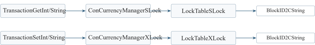
图 5-5 读写操作获取 S 锁和 X 锁的调用链
