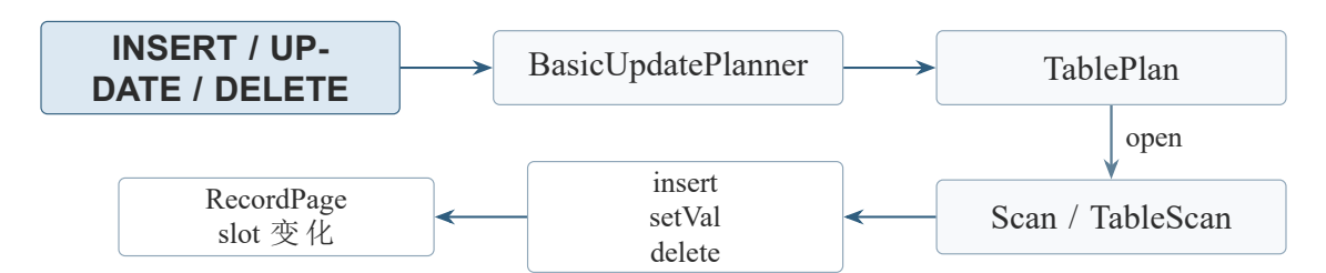
图 10-4 INSERT / UPDATE / DELETE 的记录修改链路
