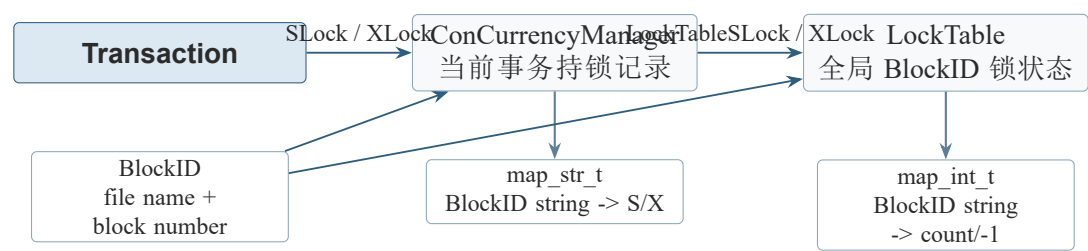
图 5-4 Transaction、ConCurrencyManager、LockTable 与 BlockID 的关系
