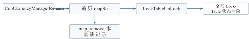
图 5-6 release all 锁释放示意图
