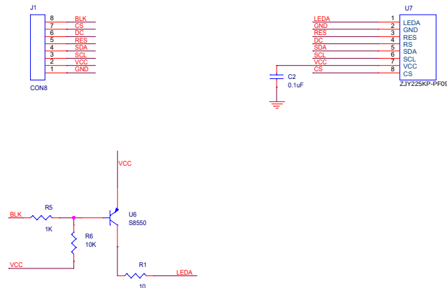
背光控制电路
