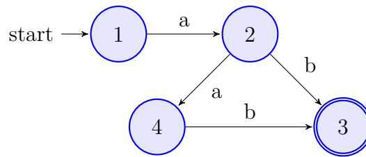
图 1: 测试 DFA 状态转换图
