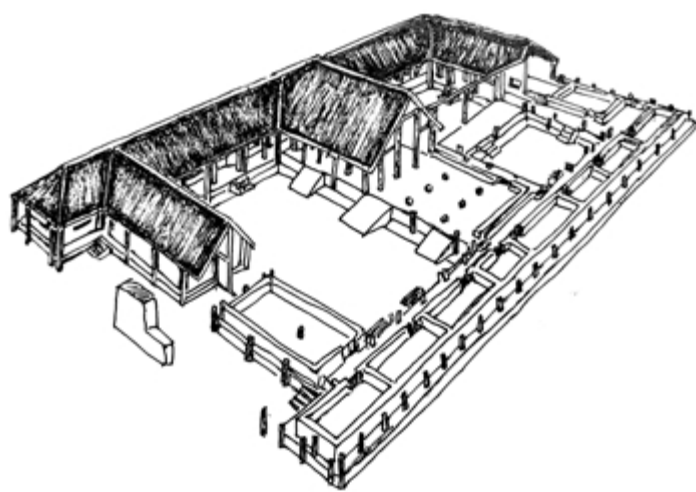
图54 岐山县凤雏村一处宫殿建筑基址
