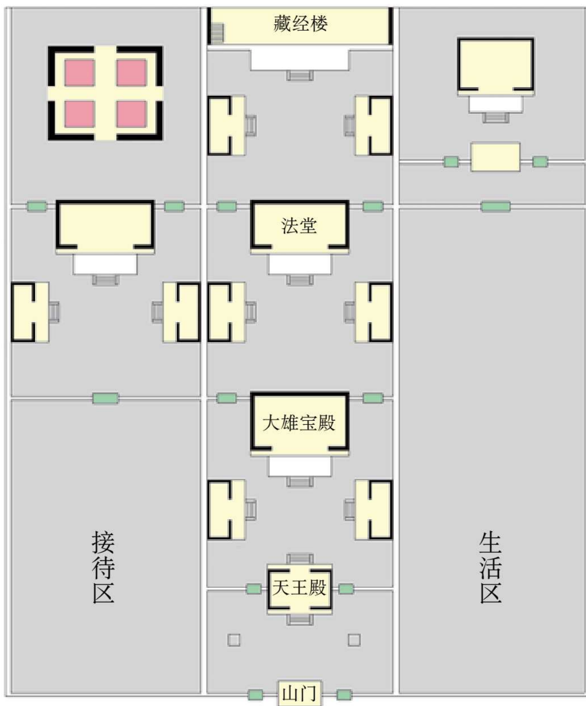
图33 汉传佛教寺院标准布局
