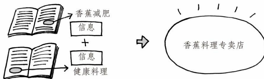
图4-2 创意的生成
