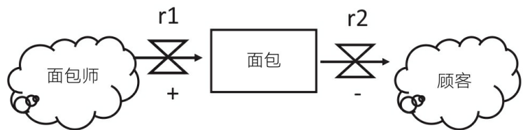
图18-2 一个关于面包店的系统动力学模型
