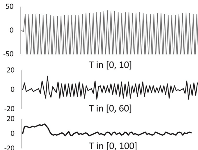
图19-6 三种阈值范围下乒乓球模型的时间序列
