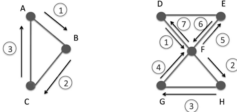
图13-2 网络上的随机游走
