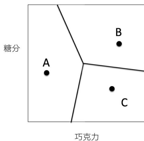
图20-4 有三种产品的空间模型（沃罗诺伊邻域）
