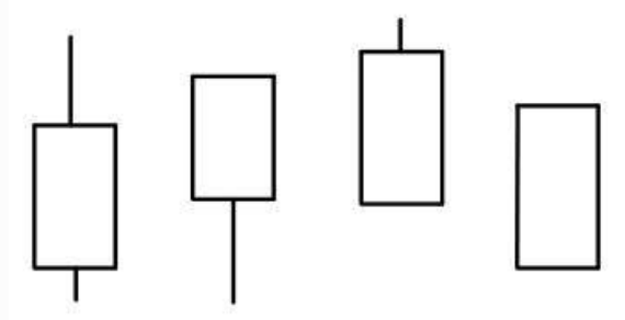
图4-21 中阳线
