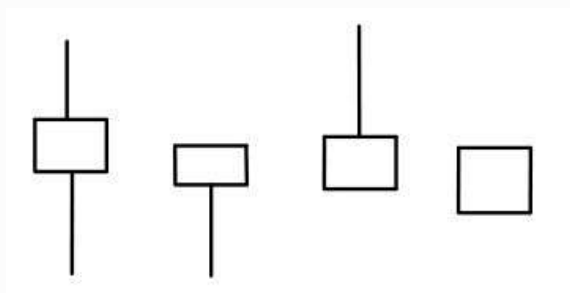
图4-23 小阳线
