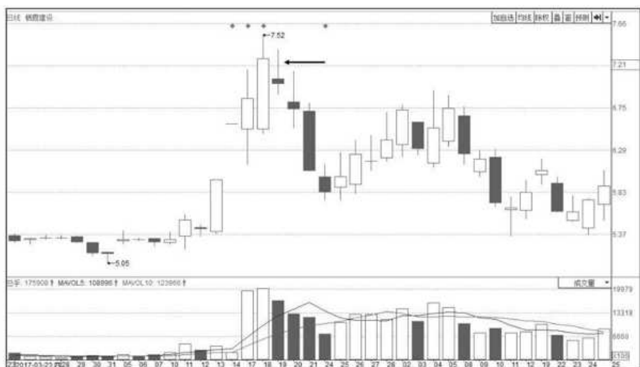
图7-15 放量见顶
