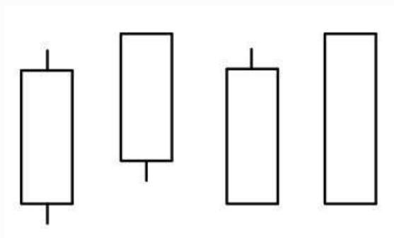
图4-18 大阳线
