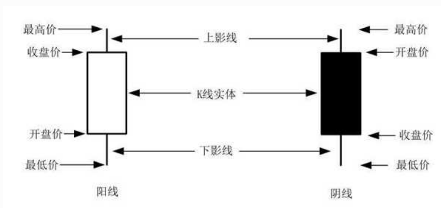
图4-7 阳线和阴线
