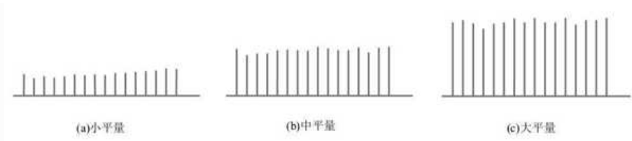
图7-11 平量示意图
