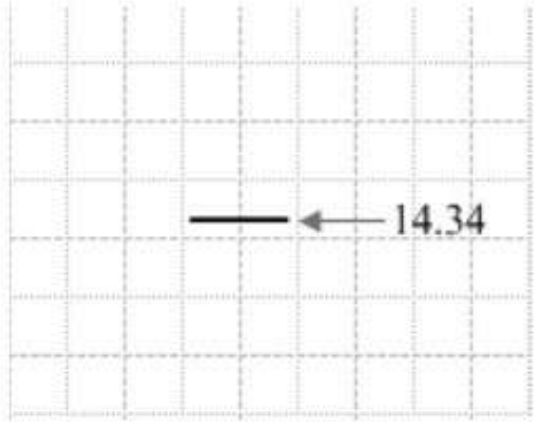
图4-9 一字K线
