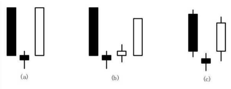
图4-25 早晨之星
