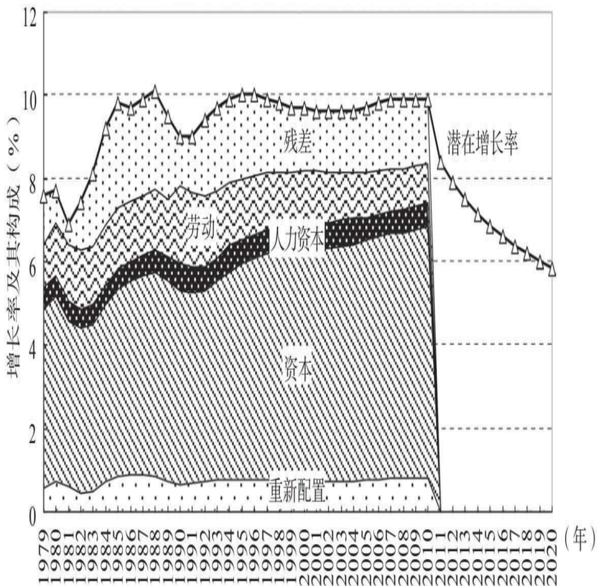
图8—1 中国经济增长的贡献因素
