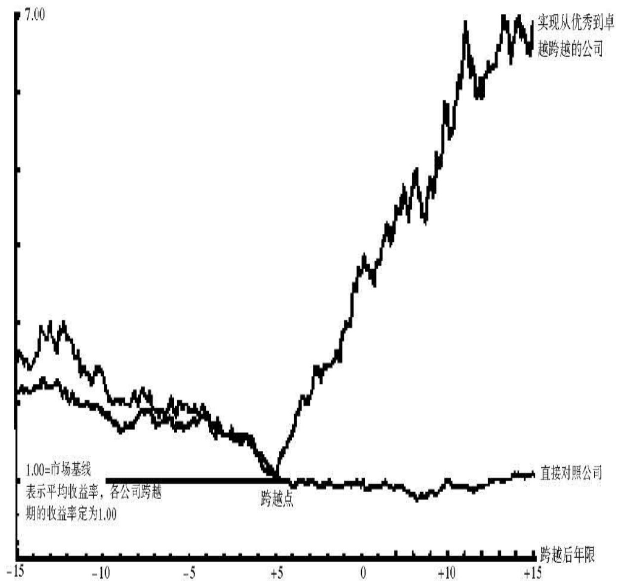
图1.1 相对于大盘股市的累积股票收益率
