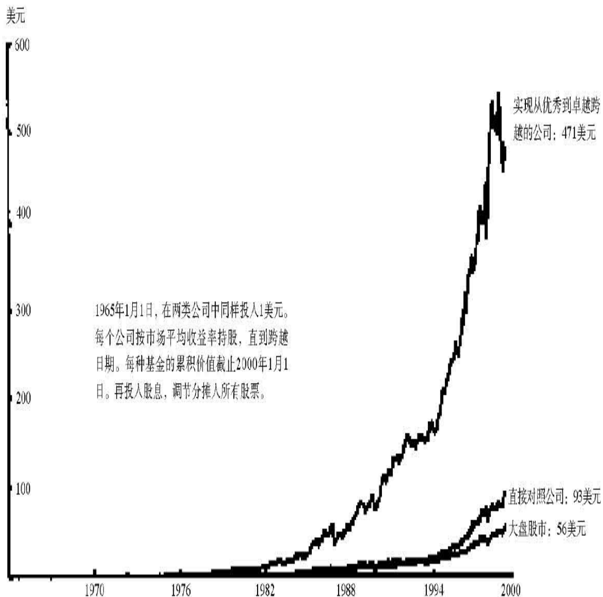
图1.2 投资1美元的累积股票收益（1965-2000）
