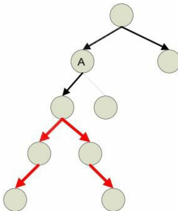
图3-14 相距最远的节点在某个子树下
