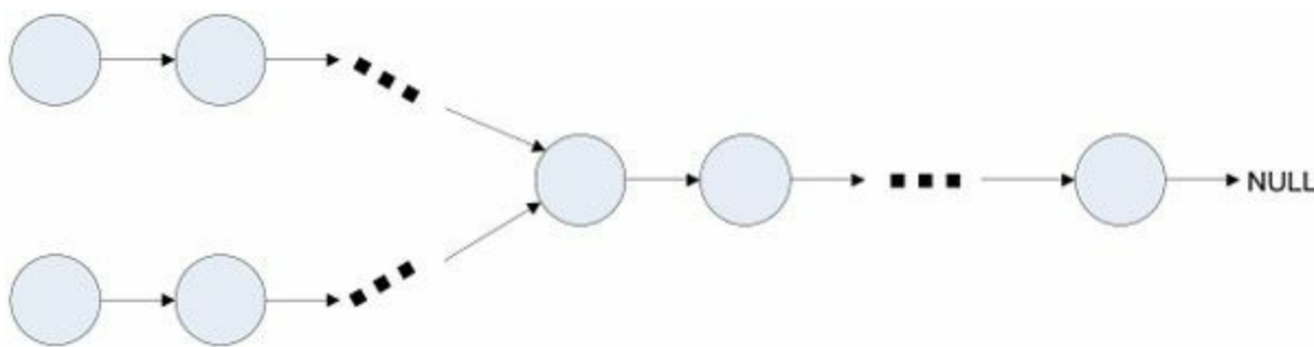
图3-8 链表相交示意图
