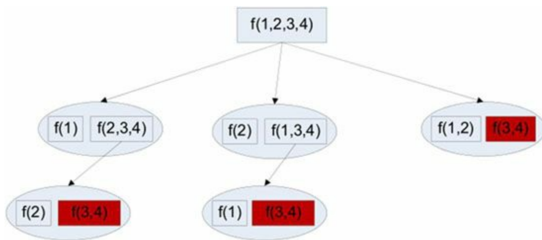
图1-26 对F函数分解示意图
