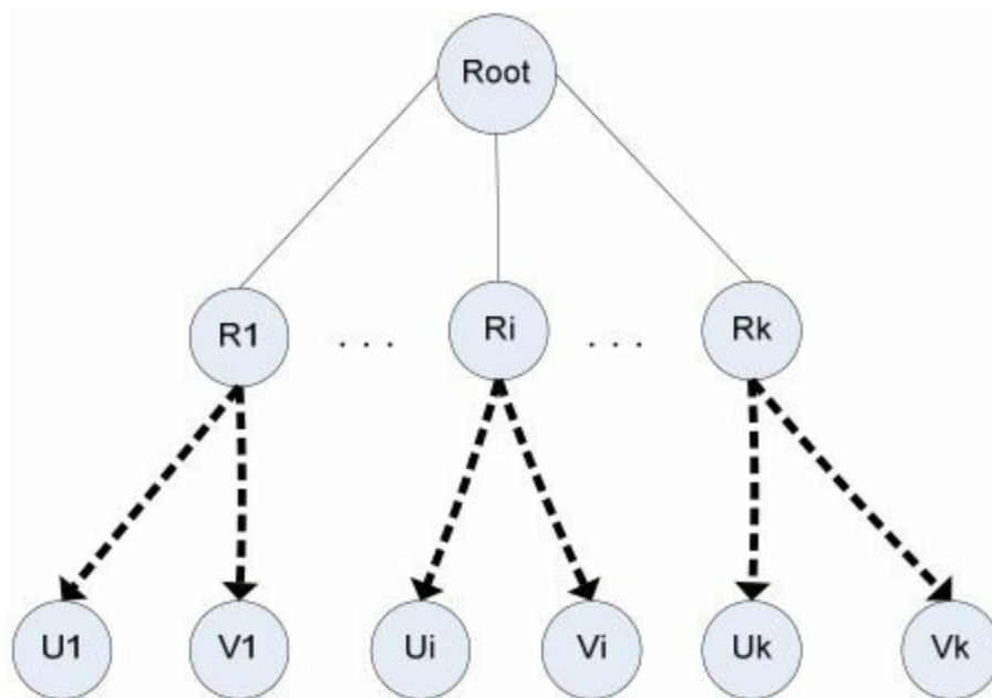
图3-15 深度遍历示意图
