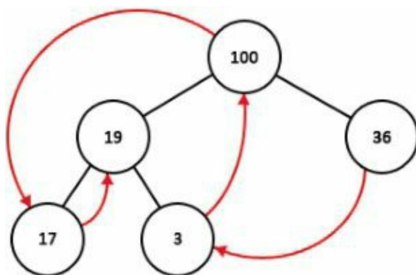
图3-10 最大堆示意图
