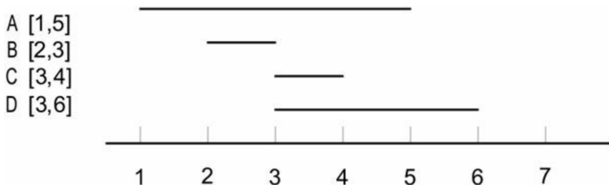
图1-14 面试时间示意图
