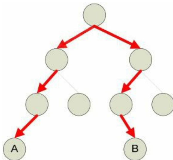
图3-11 树中相距最远的两个节点A, B
