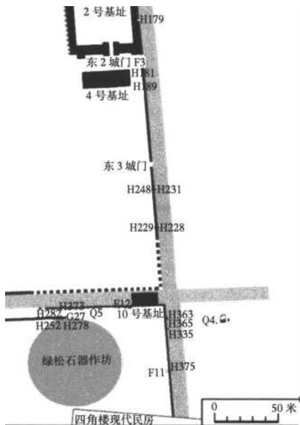
商朝占领时期的二里头宫殿区平面图8：6号和10号基址就是在这时期新建的，昔日的1号和2号基址则逐渐被废弃。
