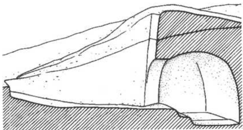
碾子坡的先周半地穴房屋和窑洞复原剖面图
