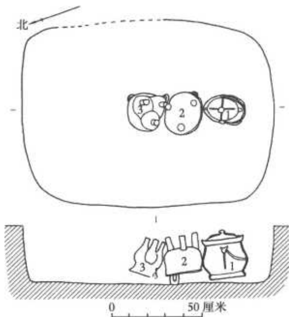
H326平面及剖面图：1. 铜提梁卤； 2, 铜鼎； 3. 铜分裆肆
