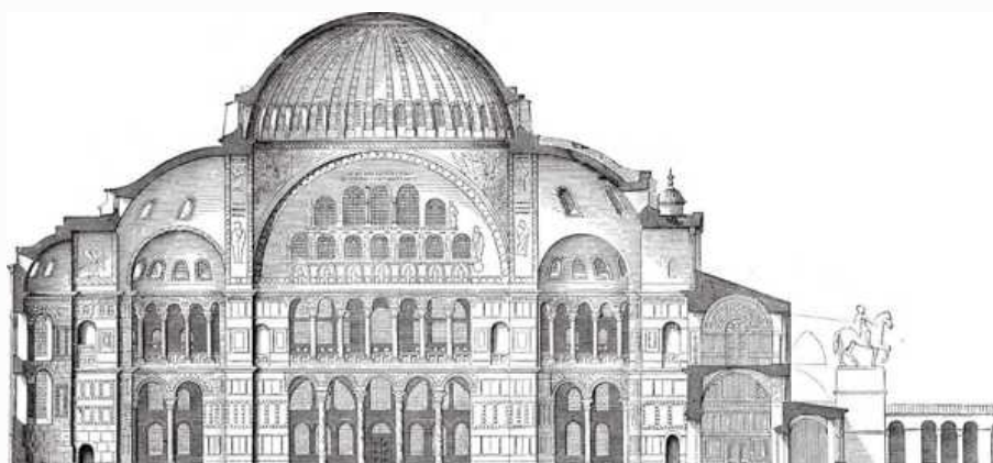
圣索非亚教堂剖面图
