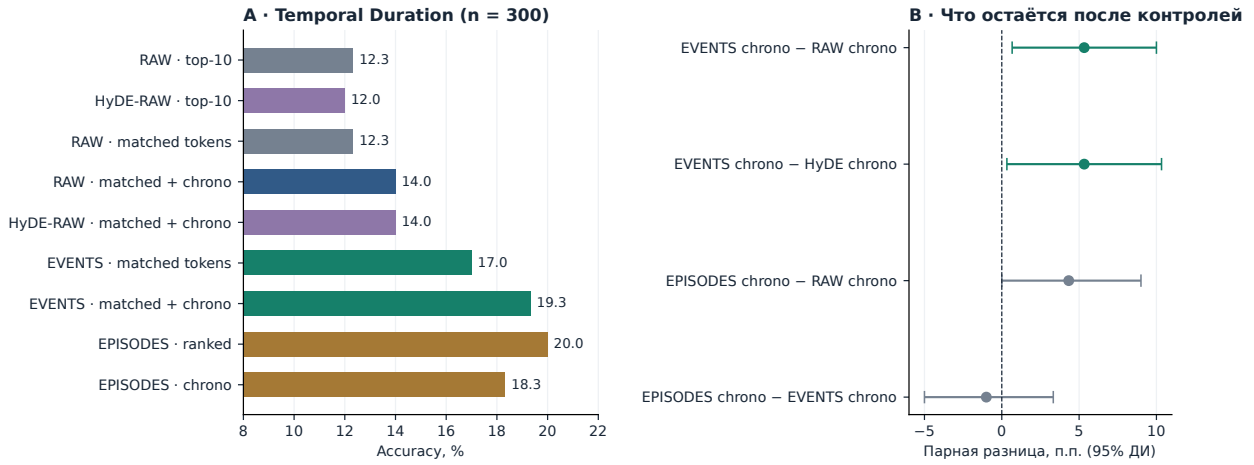
Рис. 6: Механистические контроли на exploratory Temporal Duration. EVENTS chrono сохраняют преимущество над RAW и HyDE при равном бюджете и порядке; EPISODES не превосходят EVENTS. Интервалы — question bootstrap 95%.
