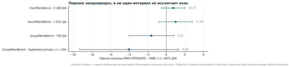
Рис. 4: Парные разницы Episodes—Raw внутри каждого набора с question- или network-bootstrap 95% ДИ. Абсолютные уровни не показаны намеренно: метрика (ассигасу против MeanQ), протоколы и answer-модели у трёх наборов различаются, и сравнивать их по высоте столбиков было бы некорректно. Group приведён после targeted repair пустых генераций; его отдельно зарегистрированный temporal/update endpoint ( n = 150 из 745) показан отдельной строкой. Ни один интервал не исключает ноль.
