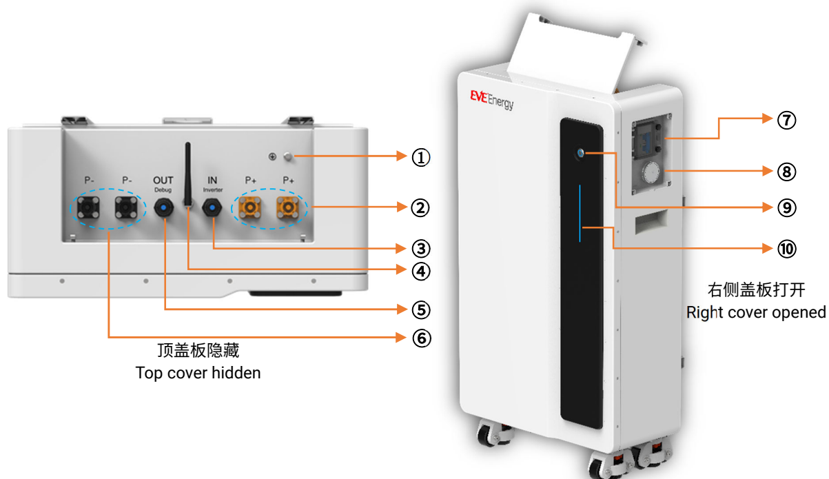
图 3 接口示意图 Figure 3 The diagram of connection terminals
