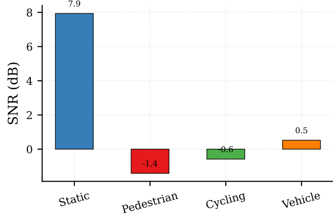
(d) Per-Scenario SNR
