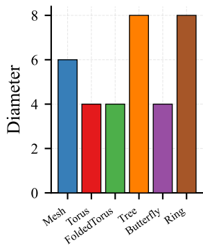
(d) Network Diameter
