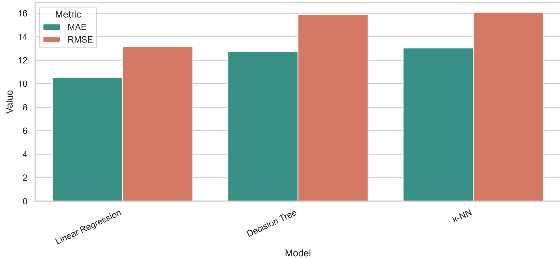
RQ1: Baseline Error Metrics
