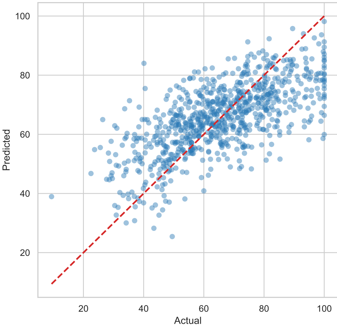
RQ2: Actual vs Predicted (Linear Regression)
