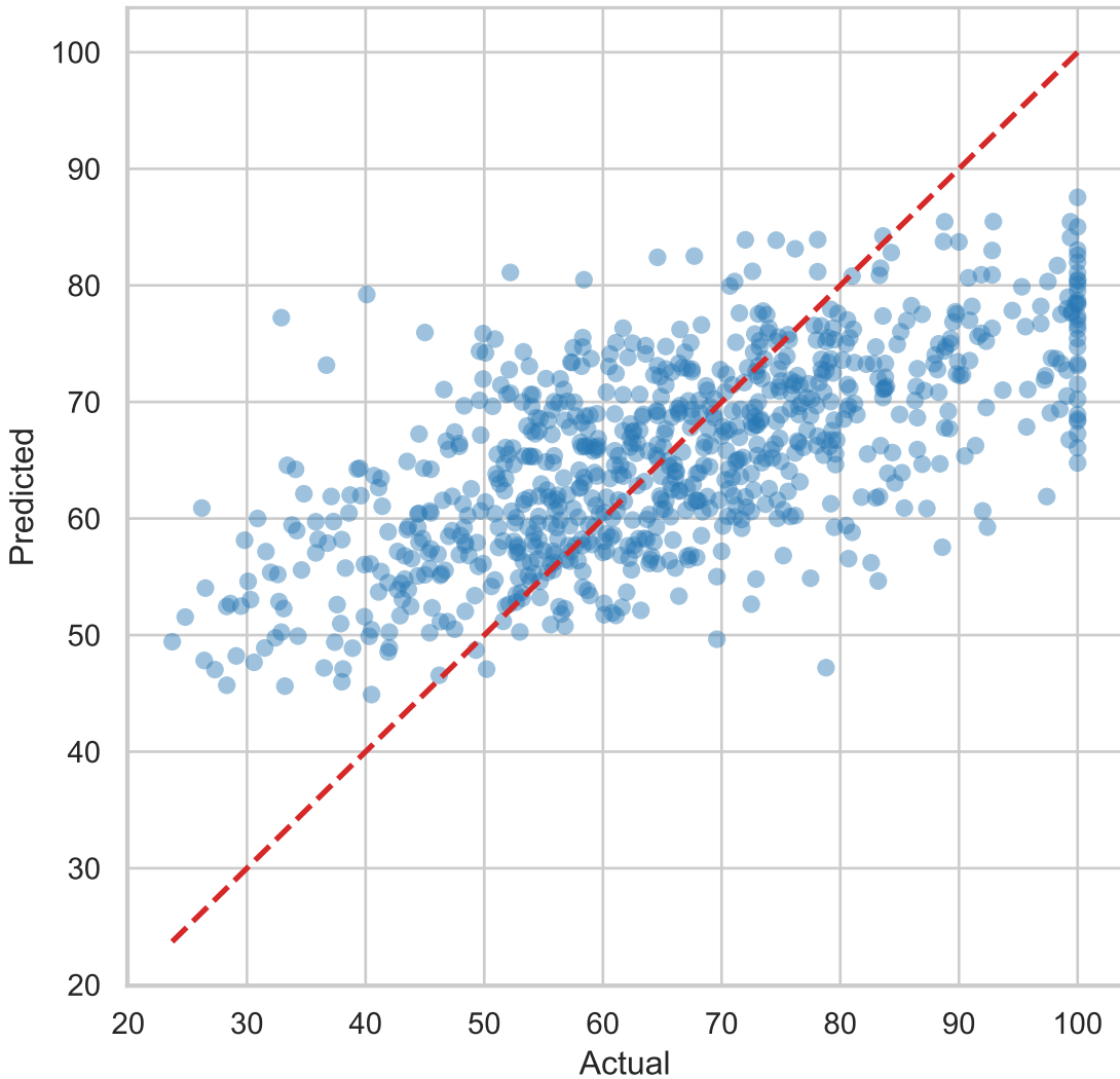
RQ4: Actual vs Predicted (Random Forest)
