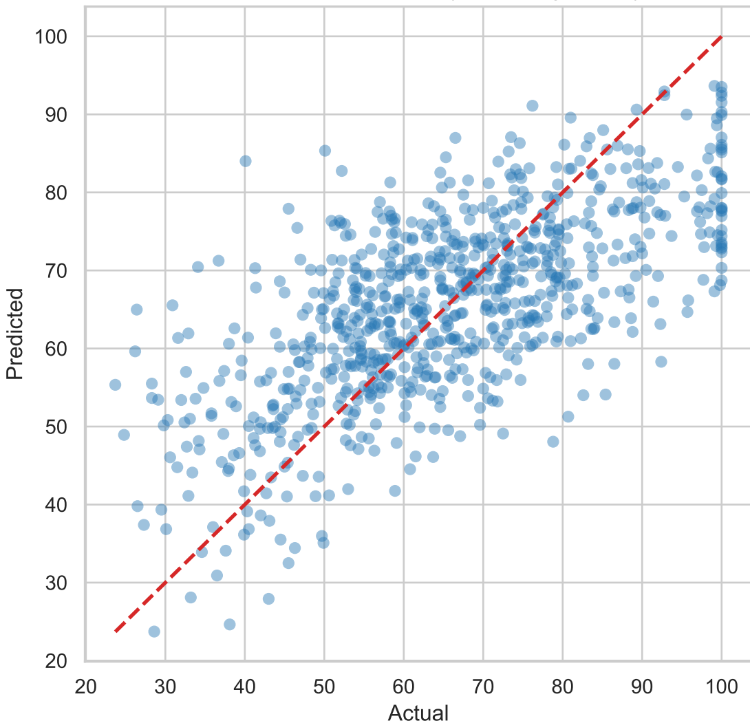
RQ7: Actual vs Predicted (Linear Regression)
