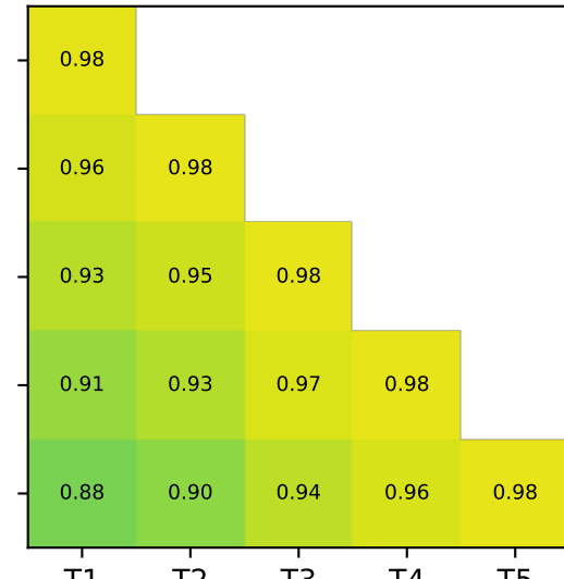
MLP + EWC
