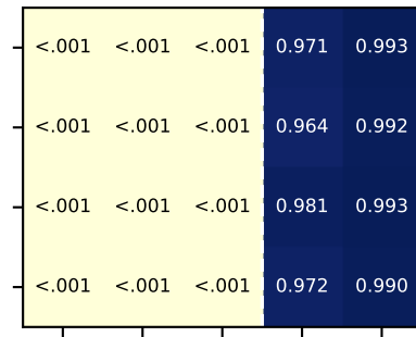
EMPIAR-10076
