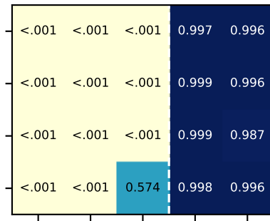
EMPIAR-10049
