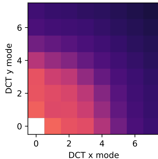
EMPIAR 10028
