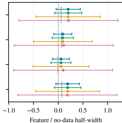
EMPIAR-10049
