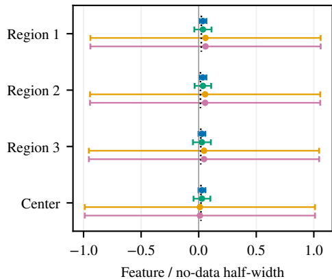
EMPIAR-10028
