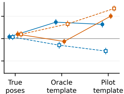
EMPIAR-10049
