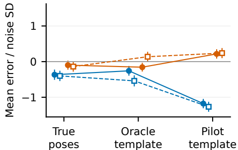
EMPIAR-10028
