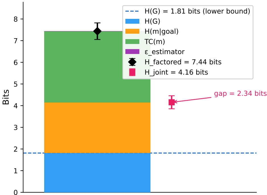
F1 — Rate Decomposition (sc_posthoc_mag, 5 seeds)
