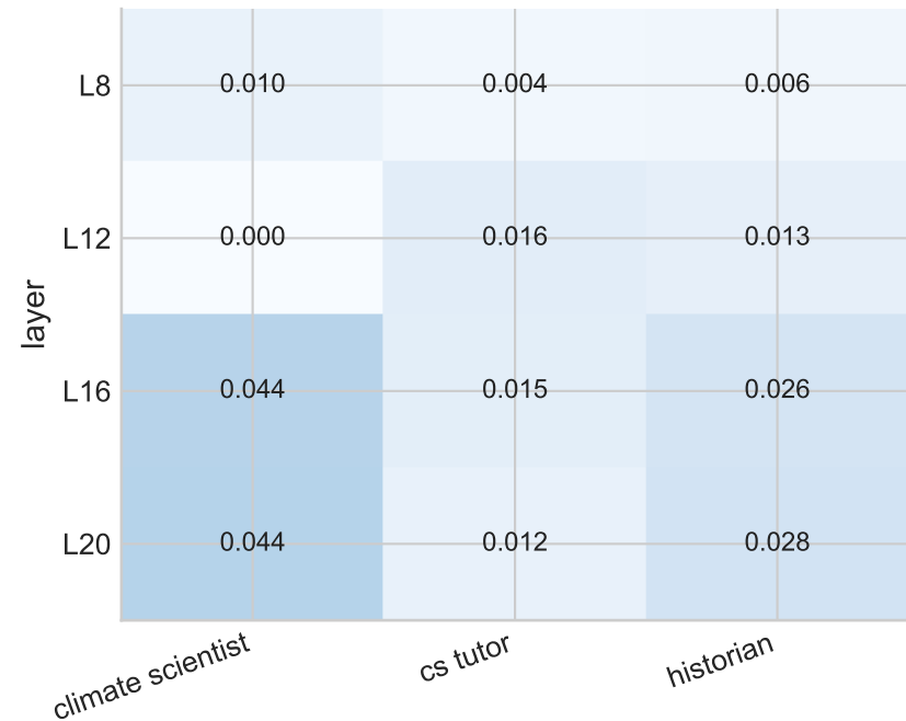
gemma2-9b-it
