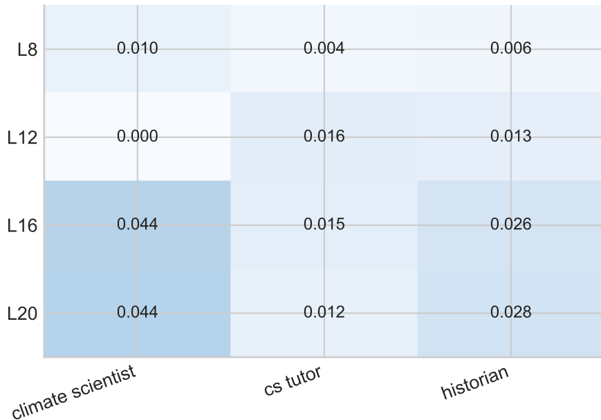
gemma2-9b-it
