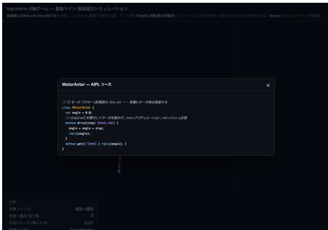
図 3: ノードをクリックすると当該アクターの AIPL ソースを表示する (図は MotorActor)。class (青)・クラス名 (橙)・文字列 (緑)・コメント (灰)に加え、Capability 注釈!{mut, net} を紫で強調。可視化が実装ソースと同期する。
