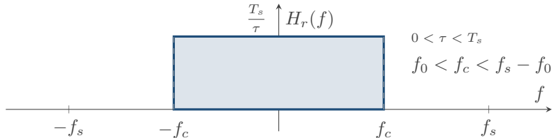
Figure 6: Filtro de reconstrução definido como pulso retangular.
