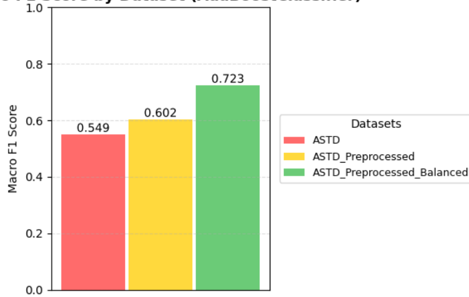
Macro F1 Score by Dataset (AdaBoostClassifier)
