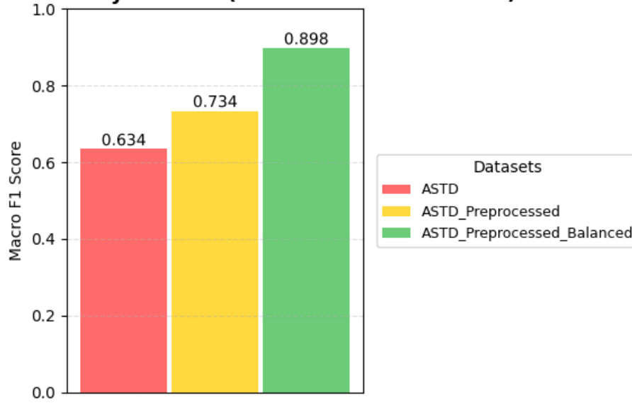
Macro F1 Score by Dataset (RandomForestClassifier)
