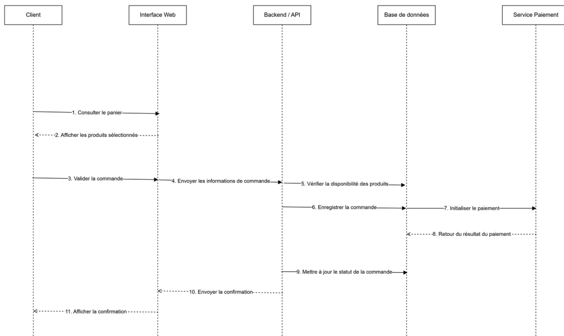
Figure 12 : Diagramme de séquence —Passer une commande
