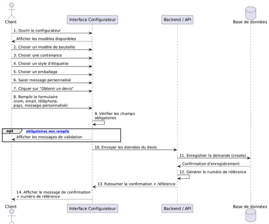
Figure 26 : Diagramme de séquence — Utiliser le configurateur
