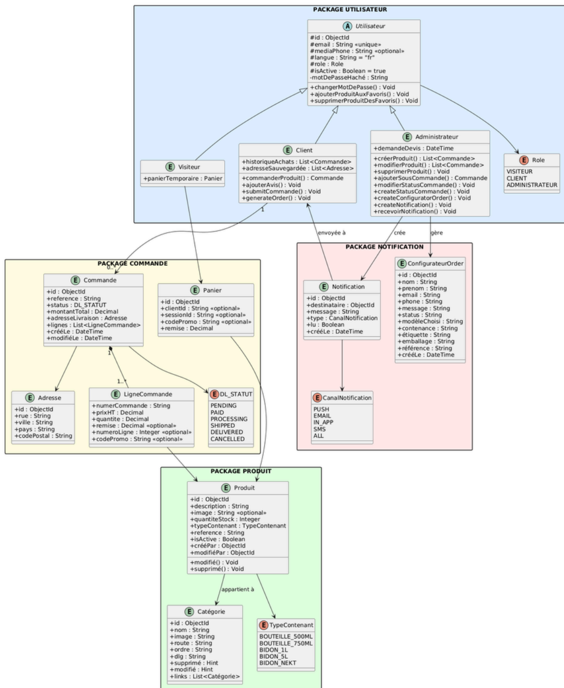
Figure 28 : Diagramme de classe
