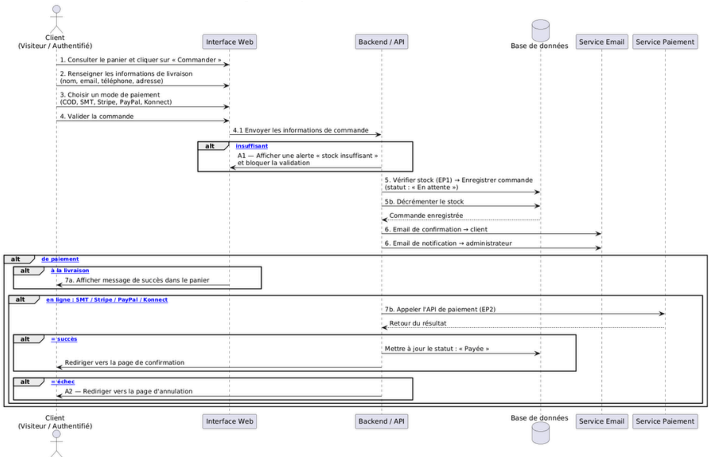
Figure 25 : Diagramme de séquence — Passer une commande
