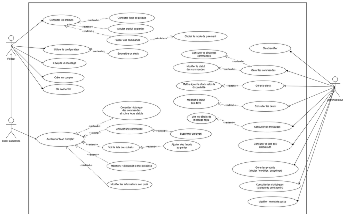
Figure 24 : Diagramme de cas d'utilisation
