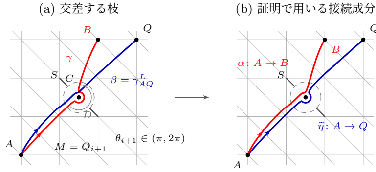
図 6.30 臨界面の配置: \epsilon = -1 , \theta_{i+1} \in (\pi, 2\pi)
