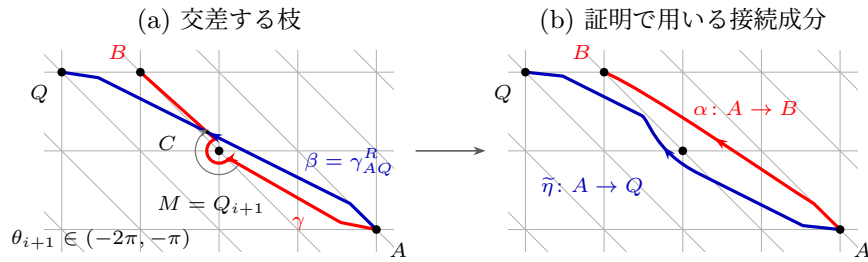
図 6.28 臨界角の配置： \epsilon = -1, \theta_{i+1} \in (-2\pi, -\pi)
