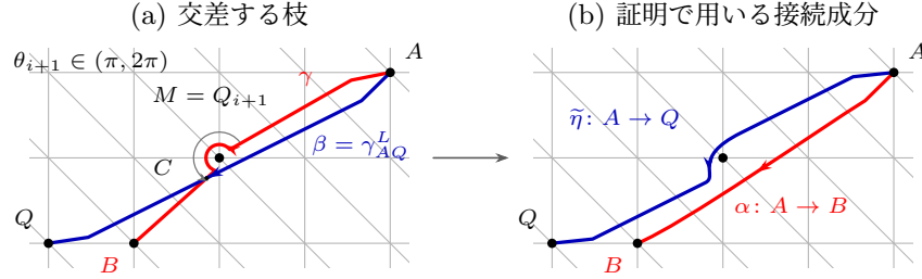
図 6.27 臨界角の配置： \epsilon = 1, \theta_{i+1} \in (\pi, 2\pi)
