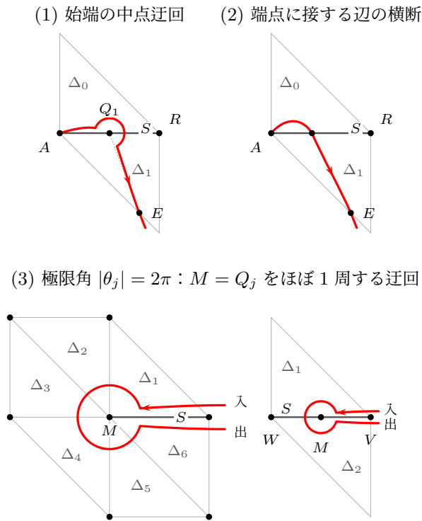
図 6.19 端点・中点付近の短縮配置
