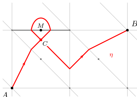
図 6.32 GM 距離を下回る自己交差弧
