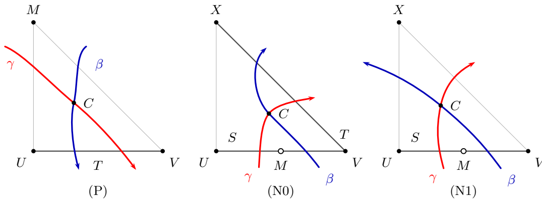
図 6.31 交差三角形 \Delta_C における (P),(N0),(N1) の配置。赤は \gamma: A \rightarrow B 、青は \beta: A \rightarrow Q を表す。
