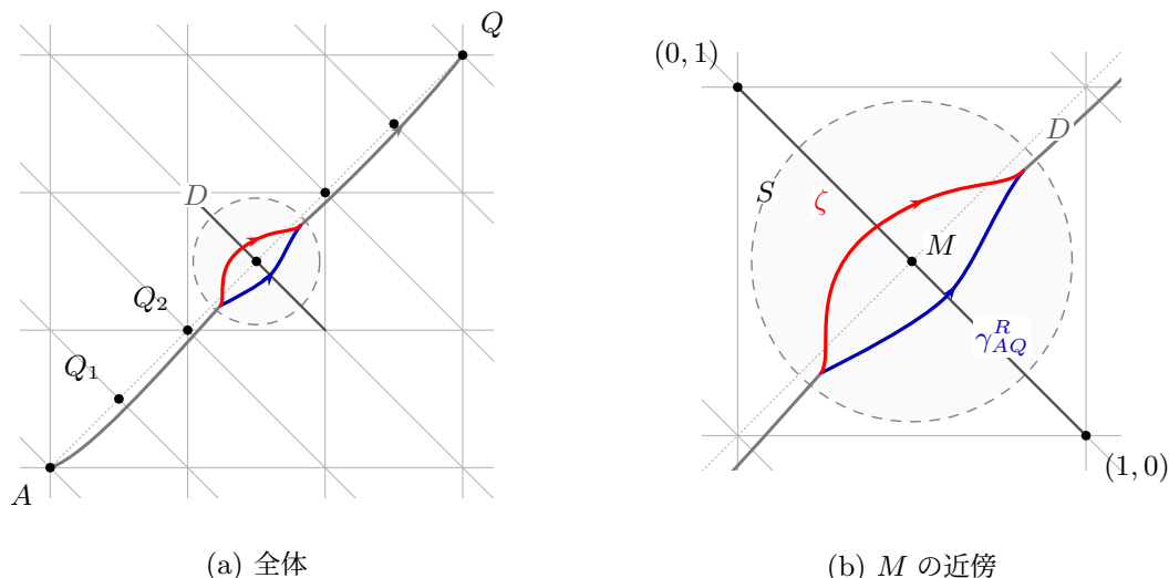
図 6.25 非格子中点での局所付替え
