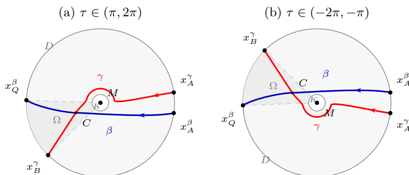
図 6.26 臨界角における円板内の交差配置
