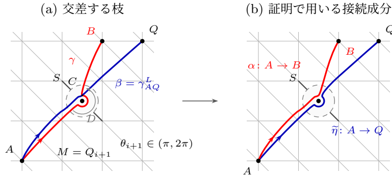
図 6.30 臨界角の配置: \epsilon = -1 , \theta_{i+1} \in (\pi, 2\pi)
