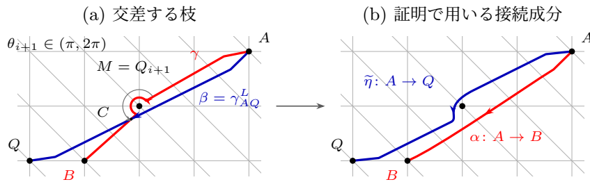
図 6.27 臨界角の配置: \epsilon = 1 , \theta_{i+1} \in (\pi, 2\pi)
