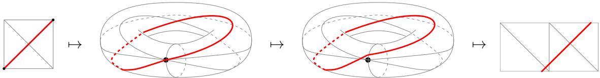
図 7.2 \overline{L}_t のトーラス上の解釈
