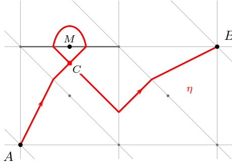
図 6.32 GM 距離を下回る自己交差弧
