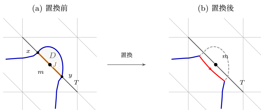
図 6.11 中点を挟む横断対の置換
