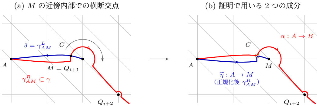
図 6.24 格子点での負の回転と局所接続
