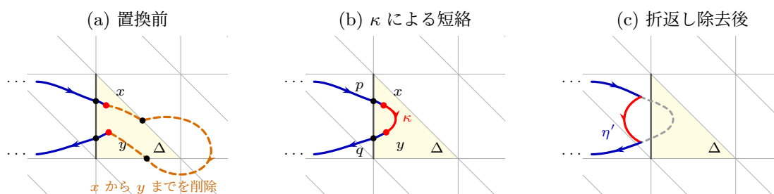
図 6.14 重複三角形の除去
