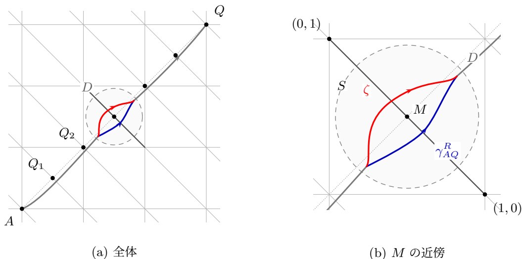
図 6.25 非格子中点での局所付替え
