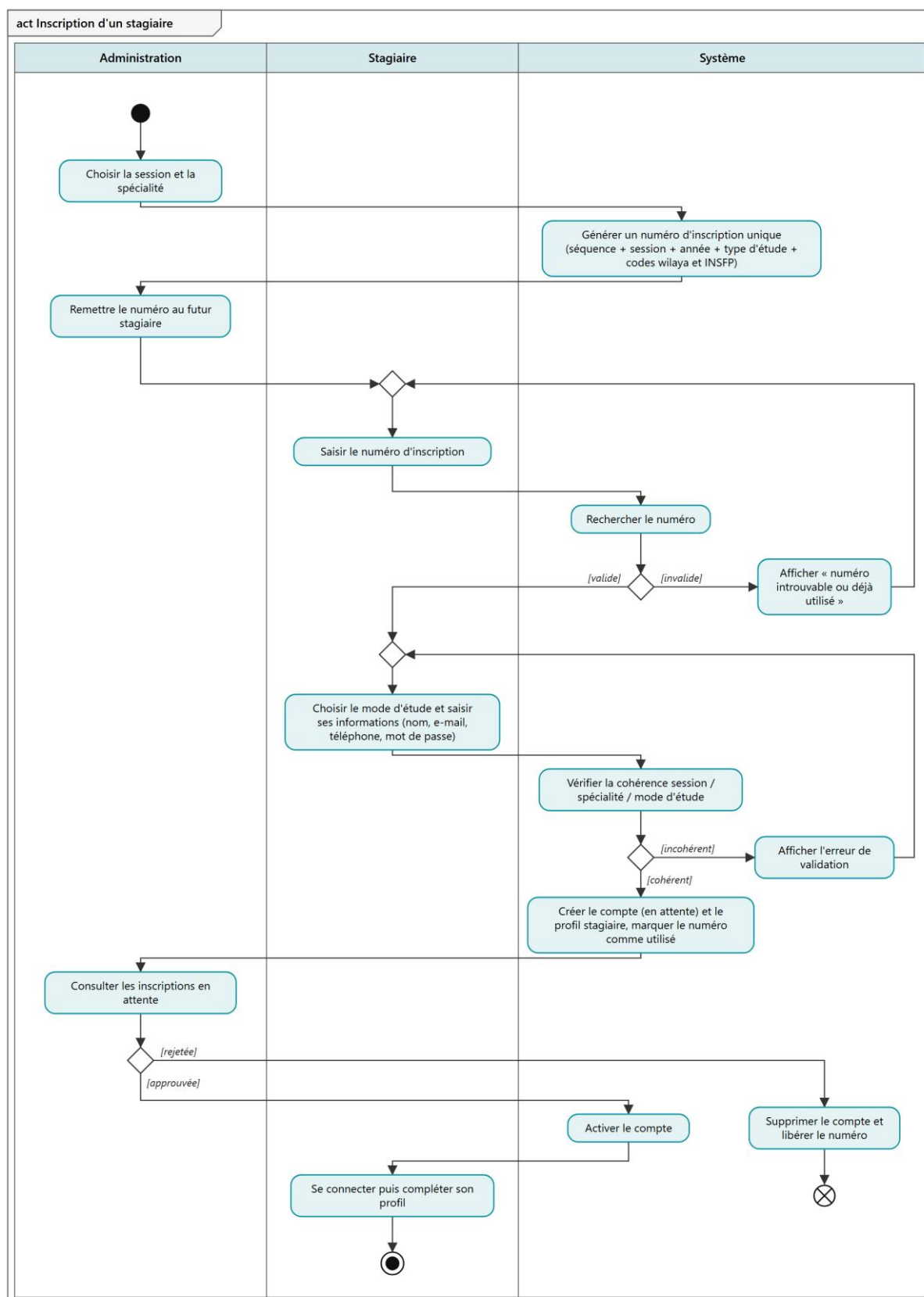
Figure 3.15 : Diagramme d'activité : inscription d'un stagiaire
