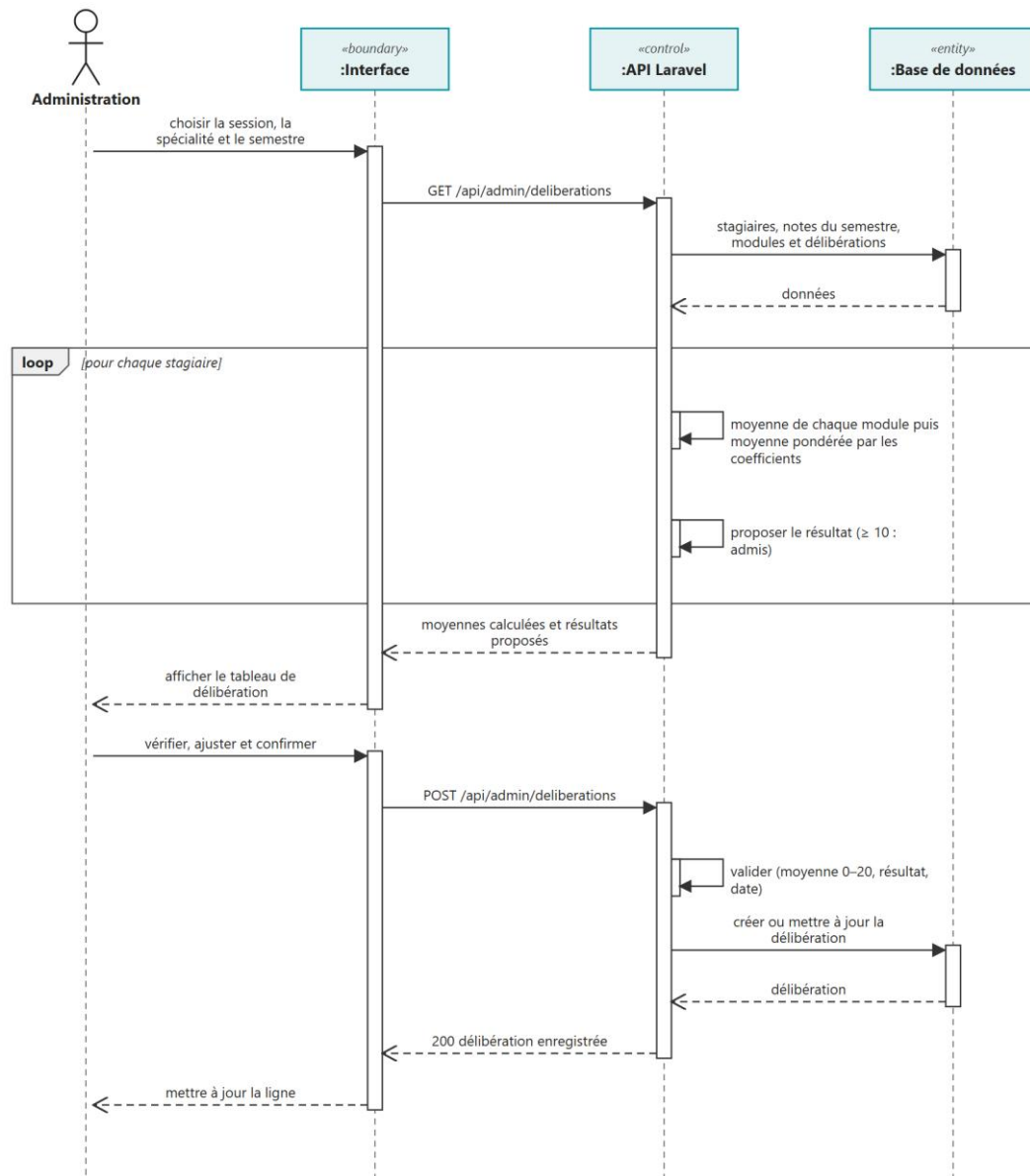
Figure 37 : Diagramme de séquence : délibération semestrielle
