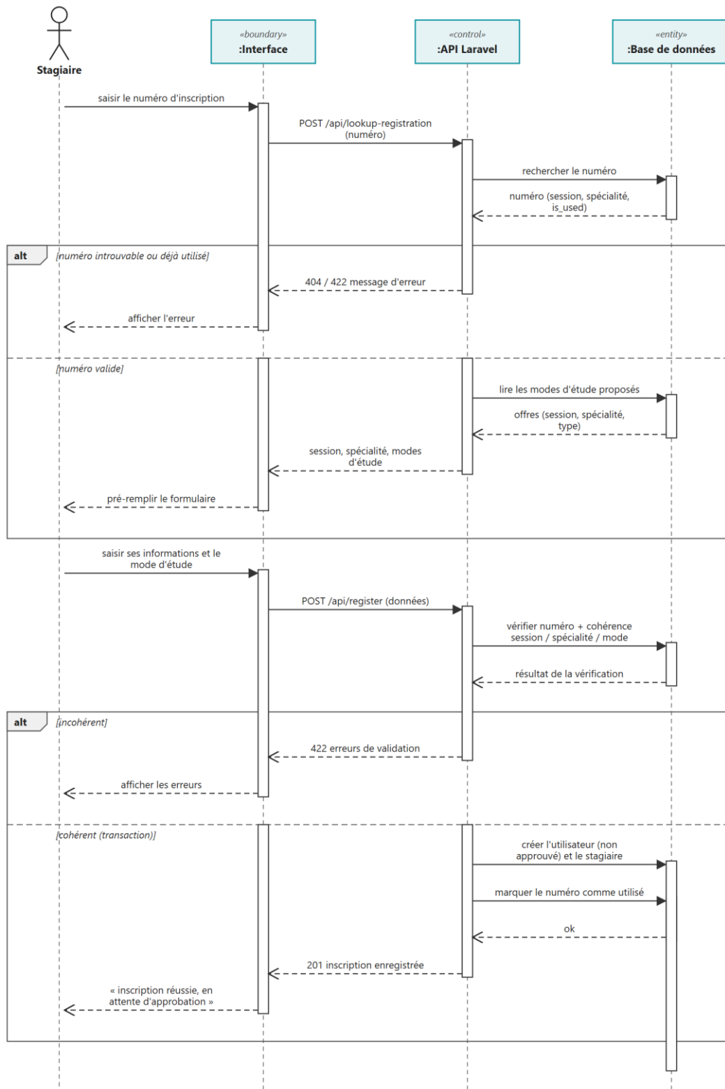
Figure 31 : Diagramme de séquence : inscription en ligne d'un stagiaire
