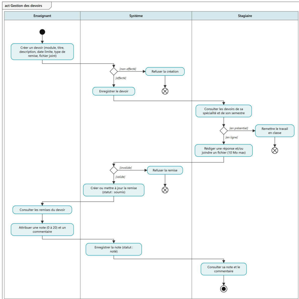
Figure 29 : Diagramme d'activité : gestion des devoirs
