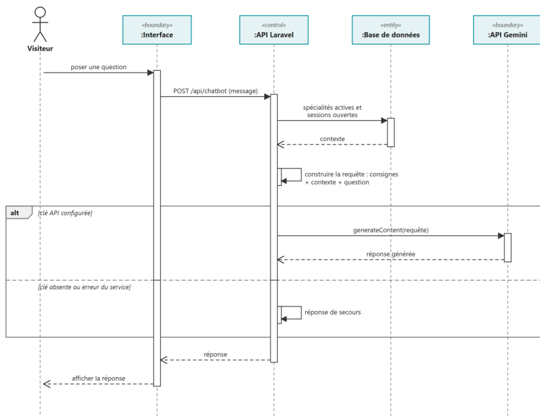
Figure 32 : Diagramme de séquence : utilisation de l'assistant intelligent
