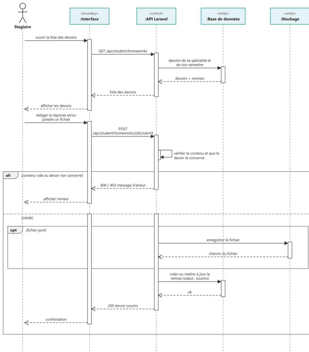
Figure 42 : Diagramme de séquence : remise d'un devoir
