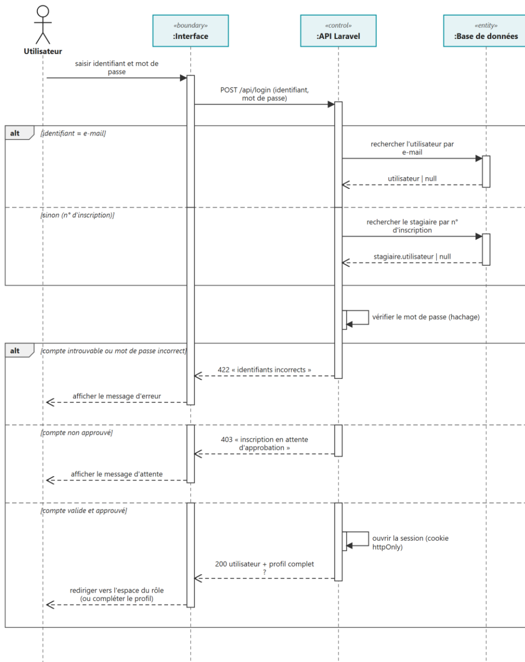
Figure 30 : Diagramme de séquence : authentification
