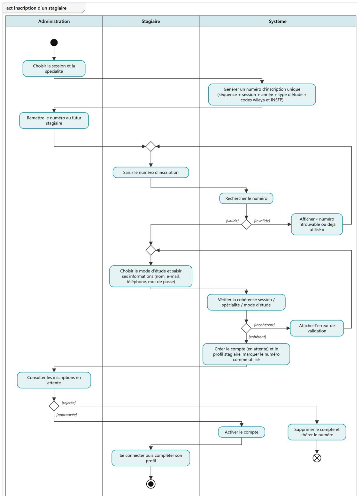
Figure 22 : Diagramme d'activité : inscription d'un stagiaire
