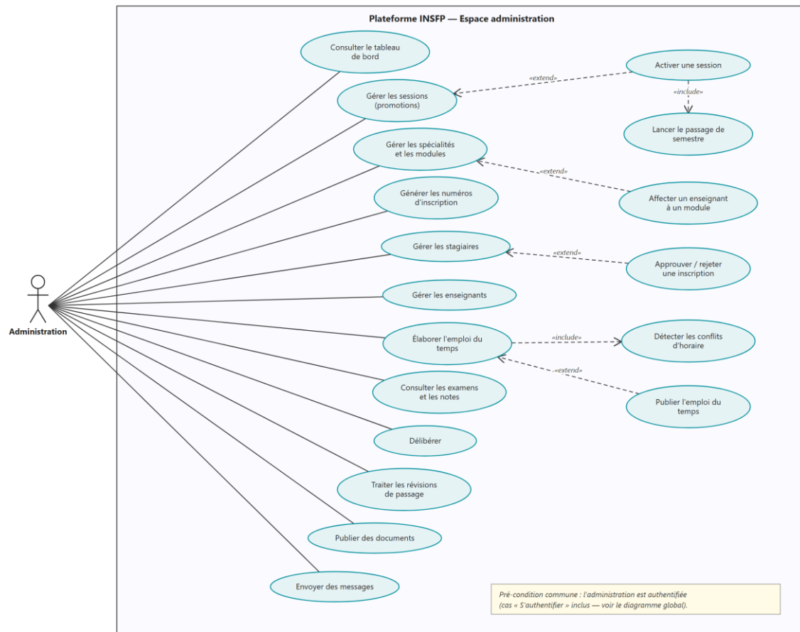
Figure 19 : Diagramme de cas d'utilisation de l'administration
