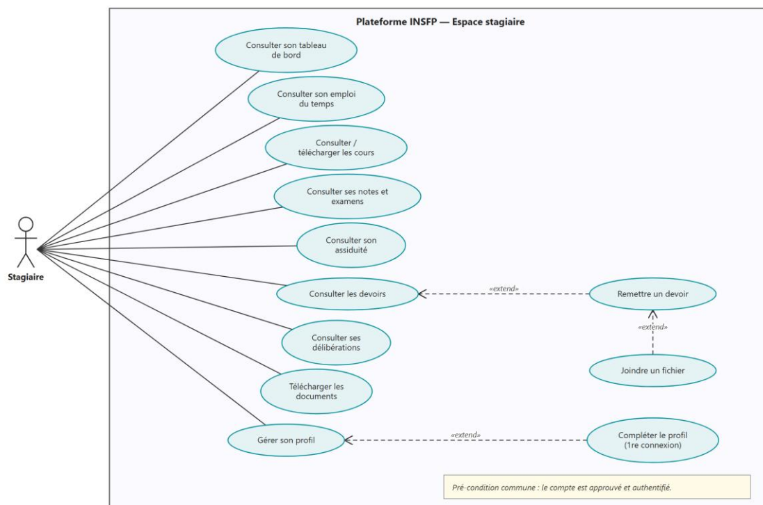
Figure 21 : Diagramme de cas d'utilisation du stagiaire
