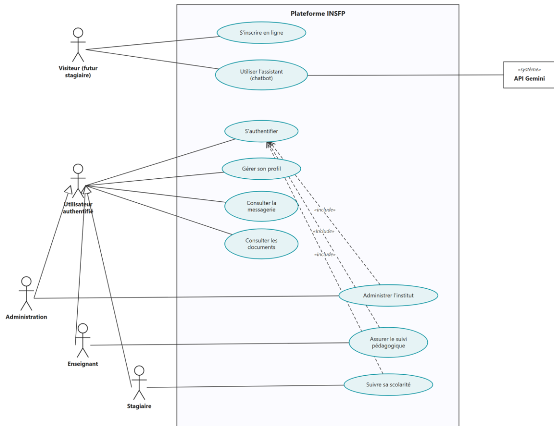
Figure 18 : Diagramme de cas d'utilisation global
