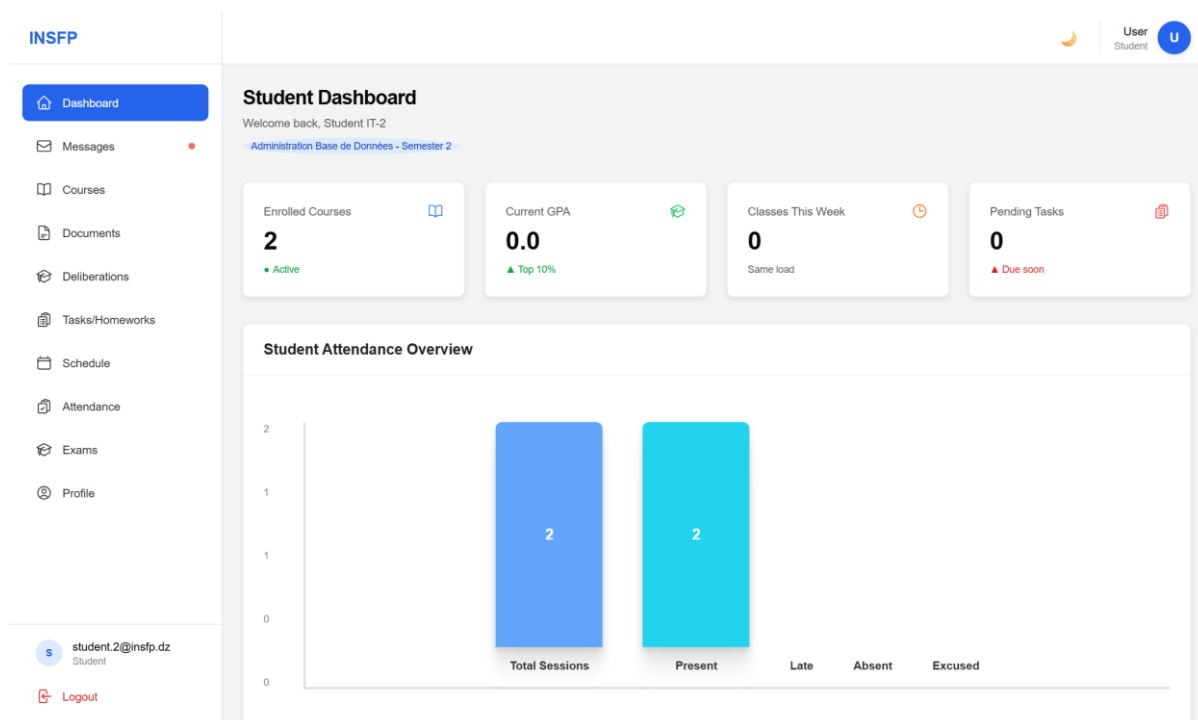
Figure 74 : Tableau de bord du stagiaire
