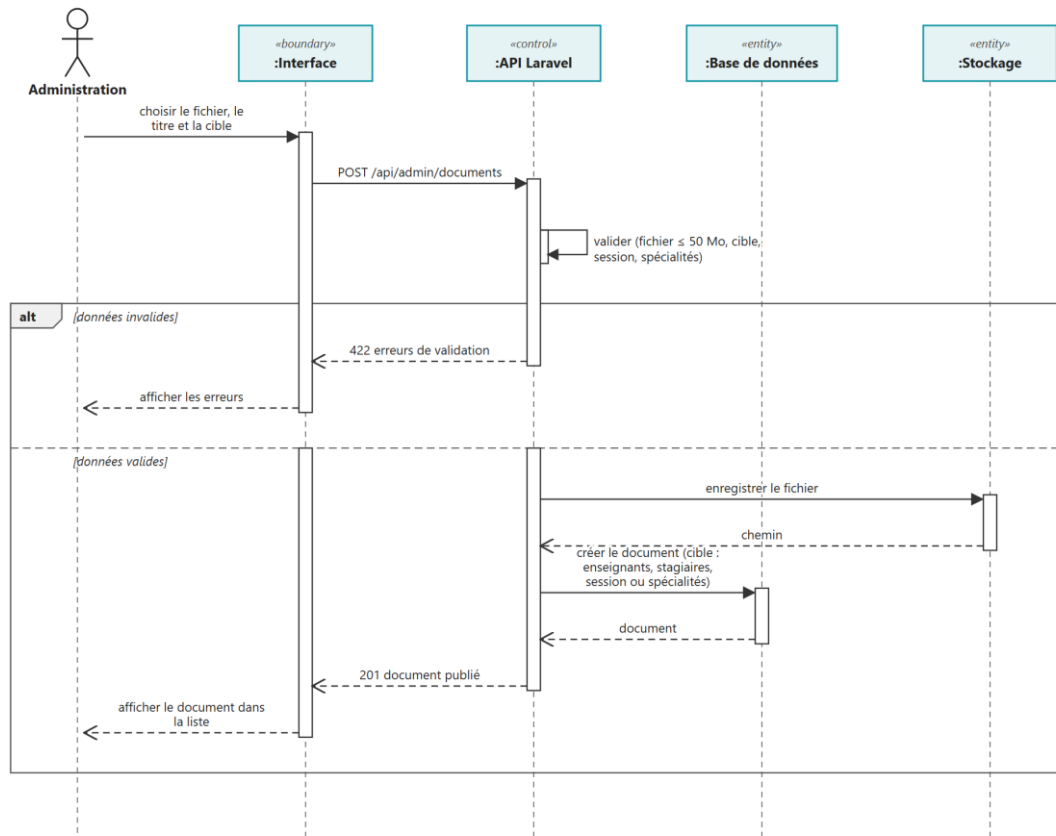
Figure 38 : Diagramme de séquence : publication d'un document
