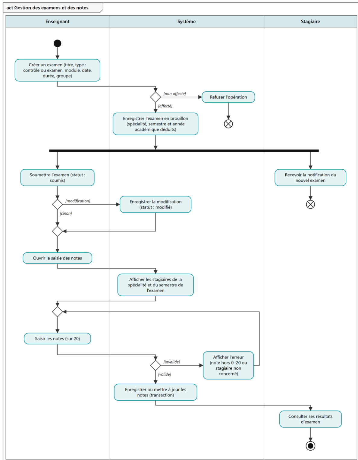
Figure 25 : Diagramme d'activité : gestion des examens et des notes
