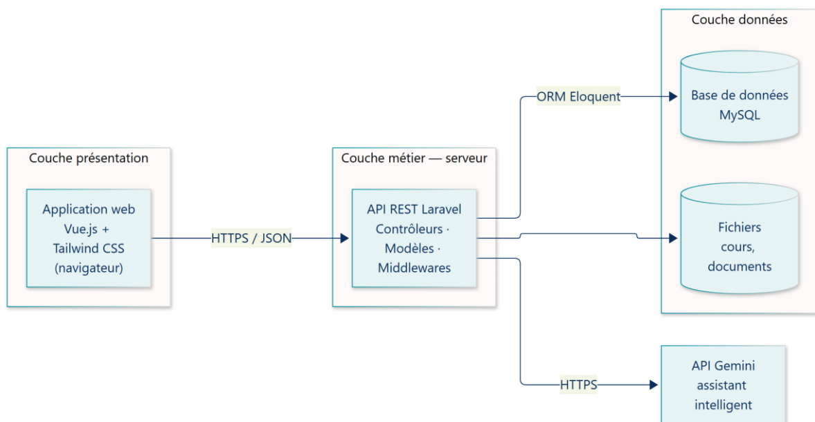
Figure 60 : Architecture trois tiers de la solution
