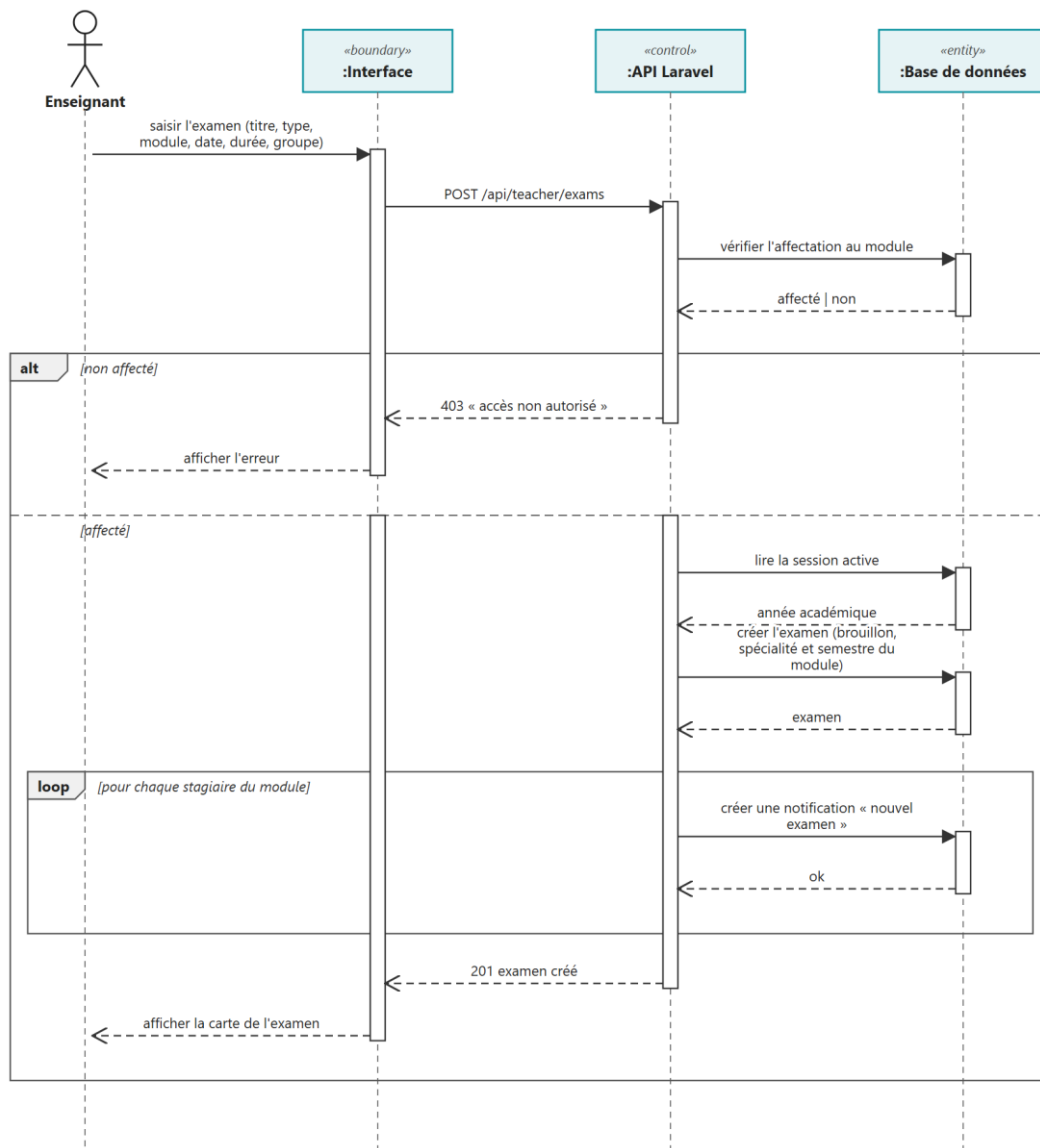
Figure 39 : Diagramme de séquence : création d'un examen
