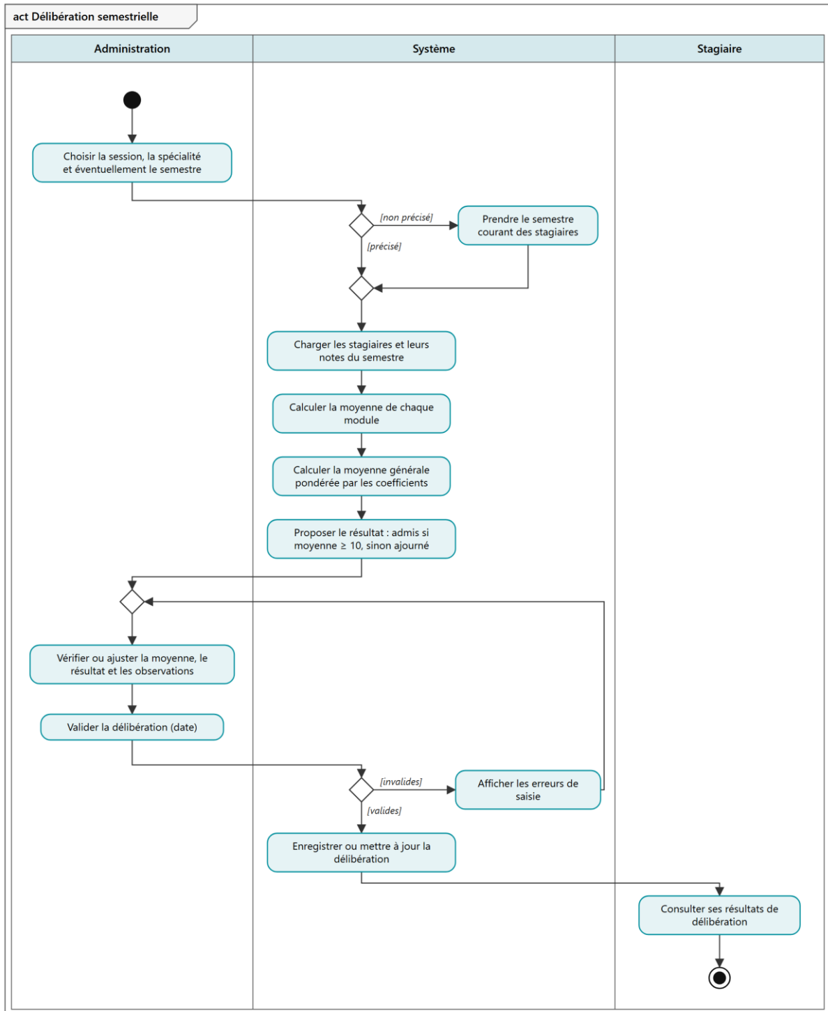
Figure 26 : Diagramme d'activité : délibération semestrielle
