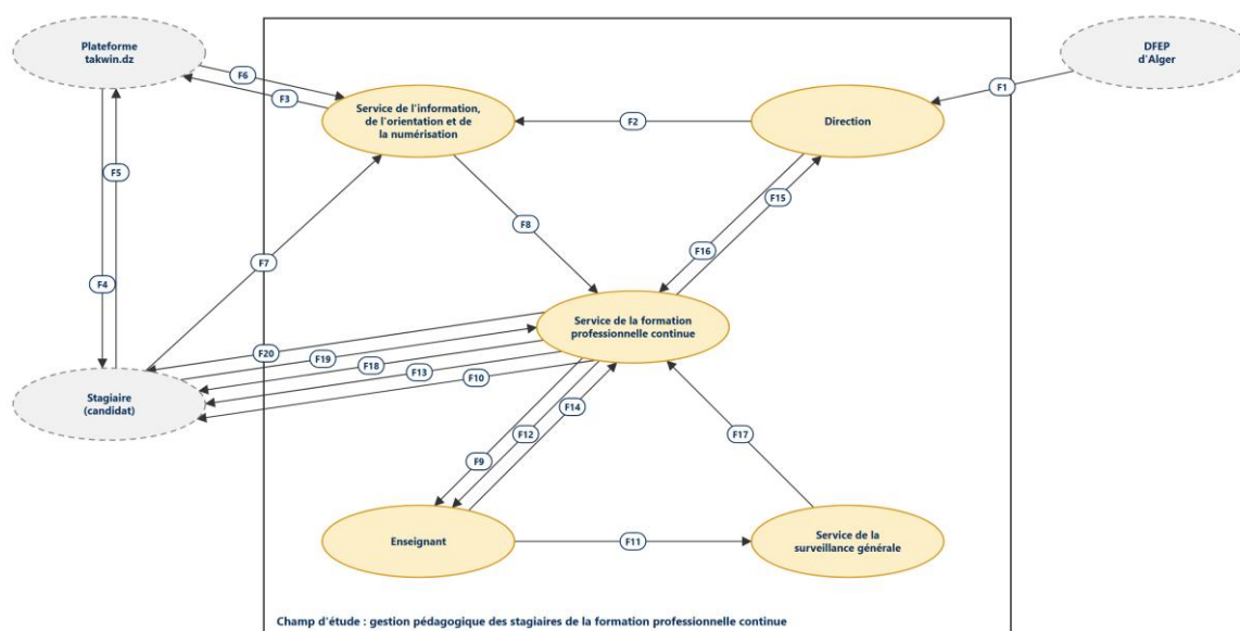
Figure 7 : Diagramme de flux d'information du système existant
