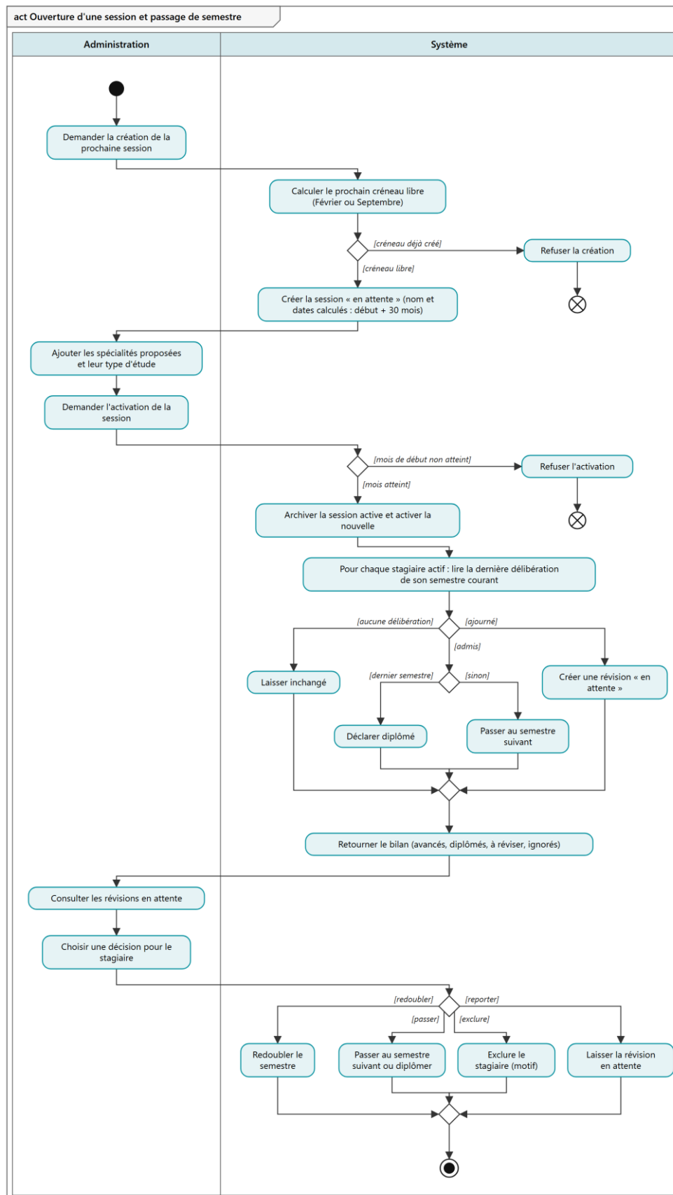
Figure 24 : Diagramme d'activité : ouverture d'une session et passage de semestre
