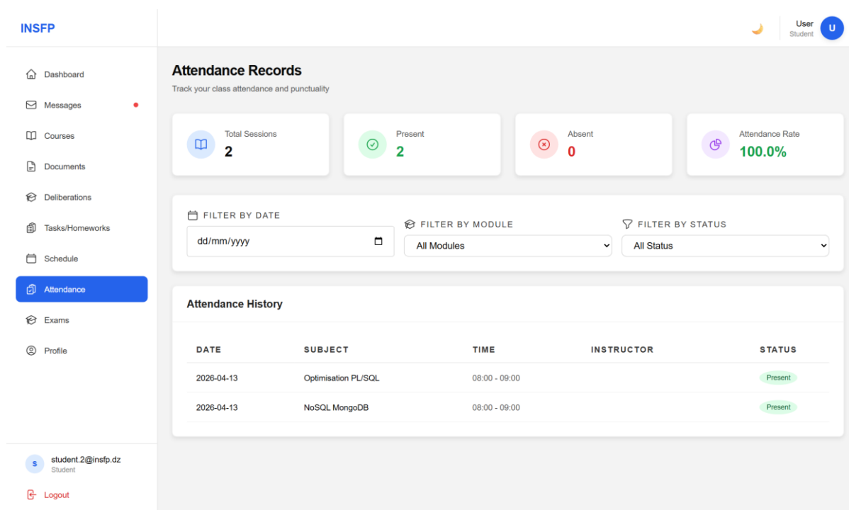
Figure 77 : Assiduité du stagiaire
