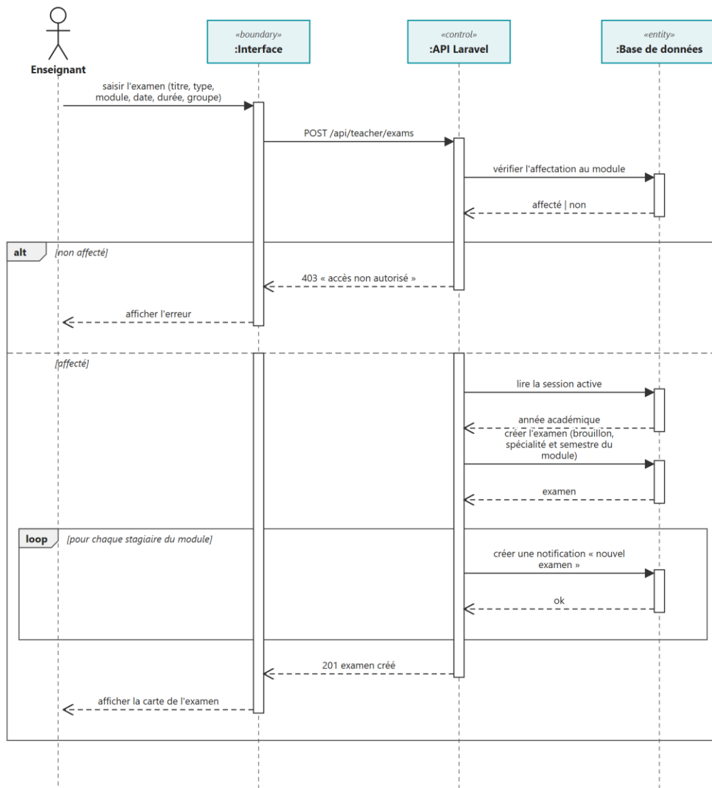
Figure 39 : Diagramme de séquence : création d'un examen
