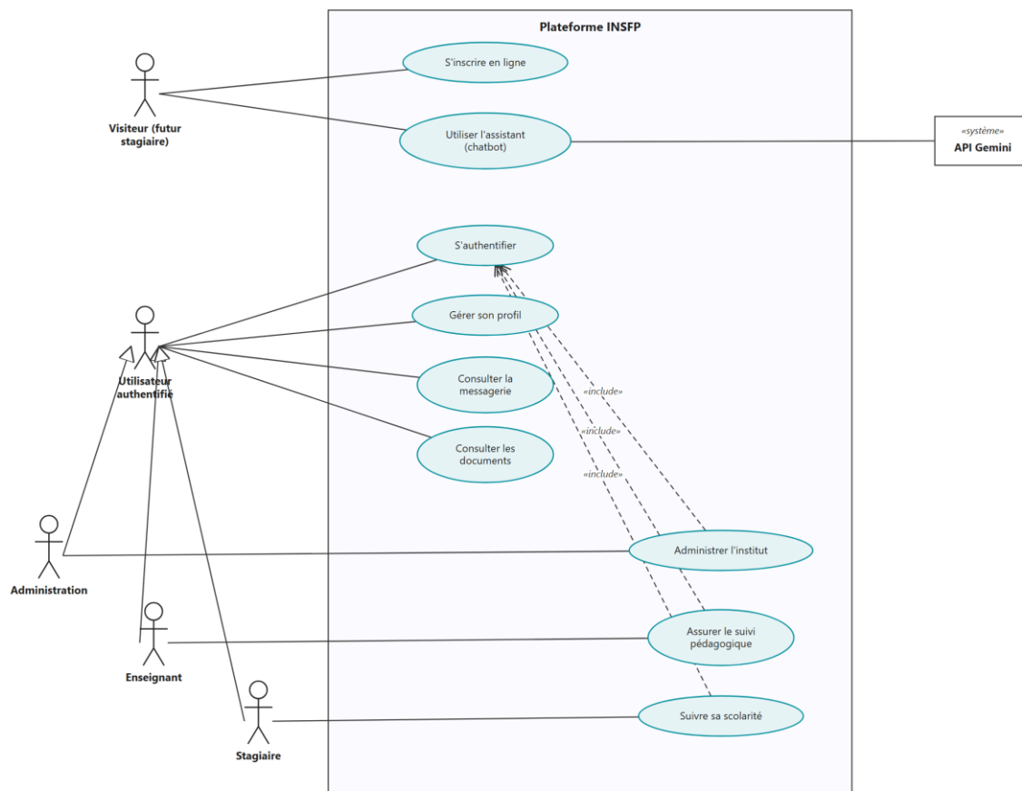
Figure 18 : Diagramme de cas d'utilisation global
