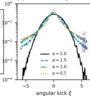
(b) \alpha -stable noise pdfs
