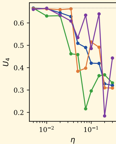
(d) U_4(\eta) , L=L_{\max}
