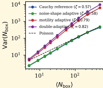
(d) number fluctuations
