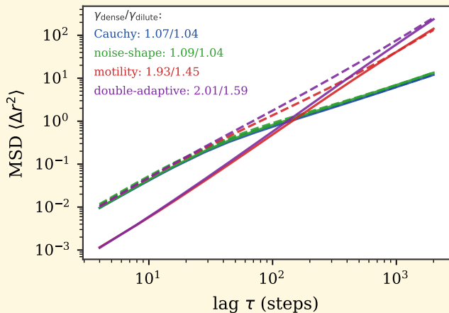
(d) stratified MSD
