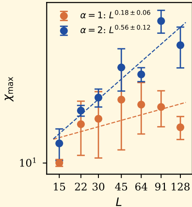
(d) FSS of \chi_{\max}
