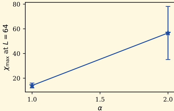
(d) FSS susceptibility peak
