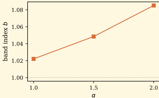
(d) FSS susceptibility peak
