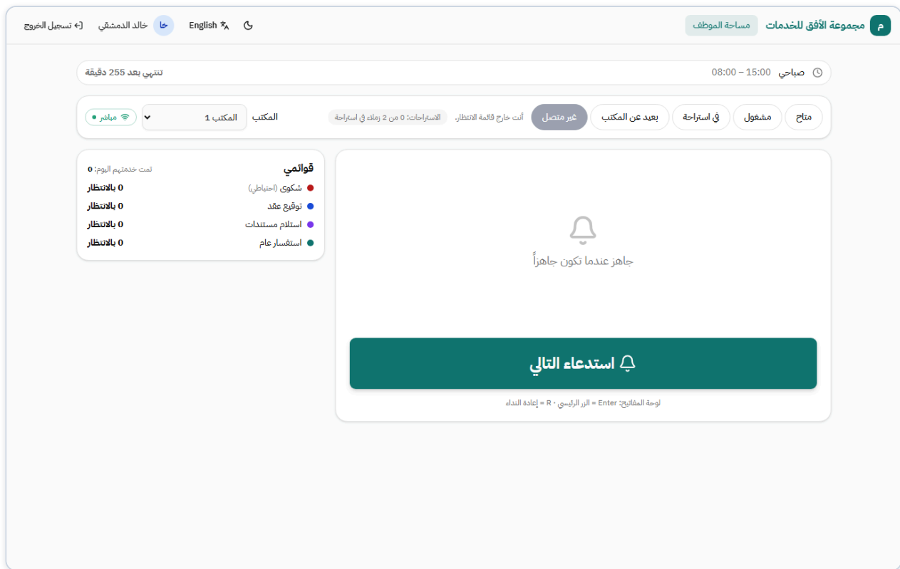
مساحة الموظف
