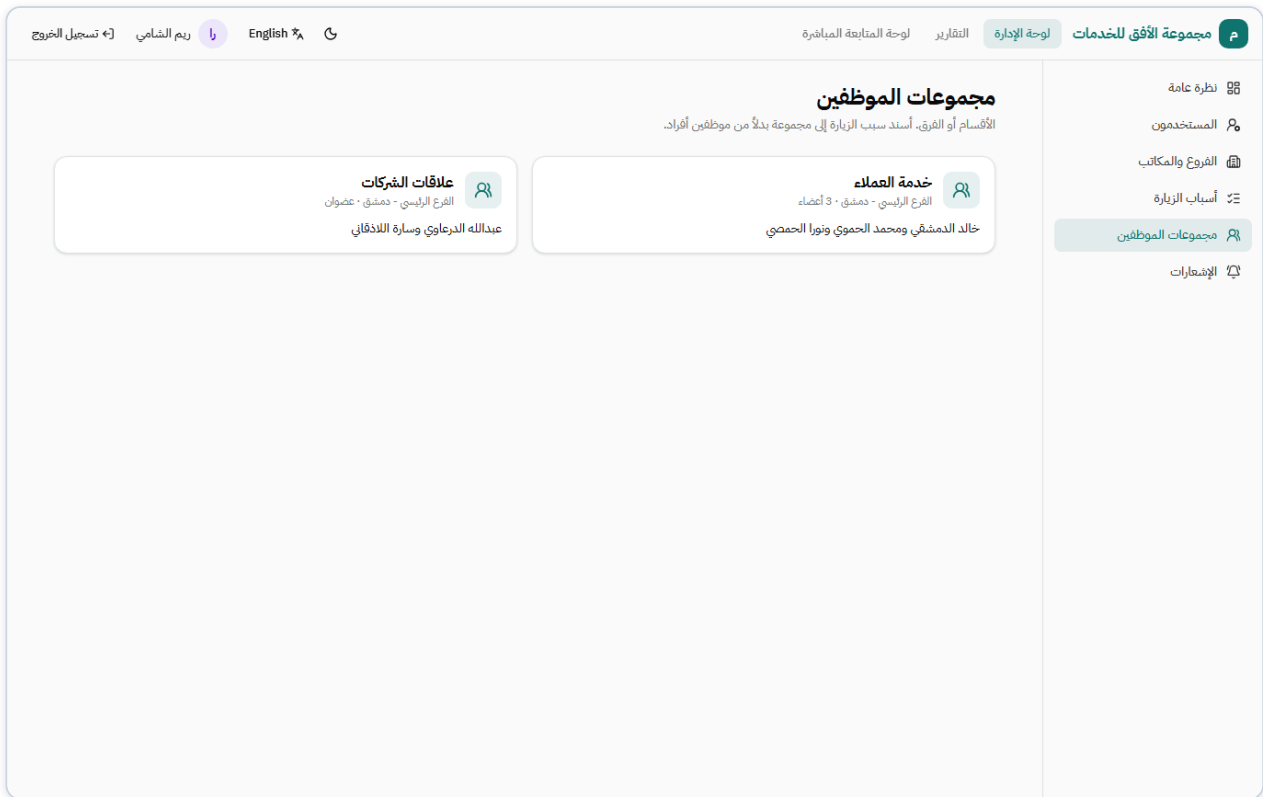
مجموعات الموظفين
