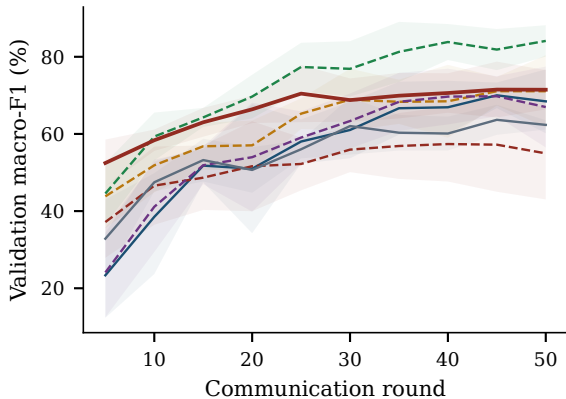
Edge-IIoTset
