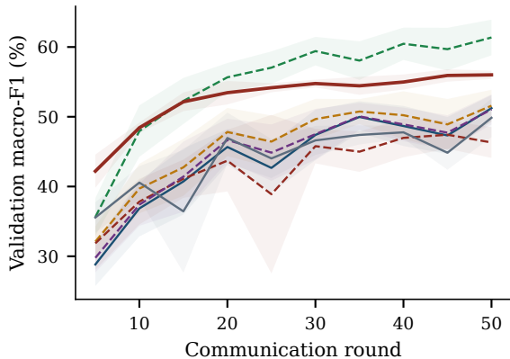
CICIoT2023
