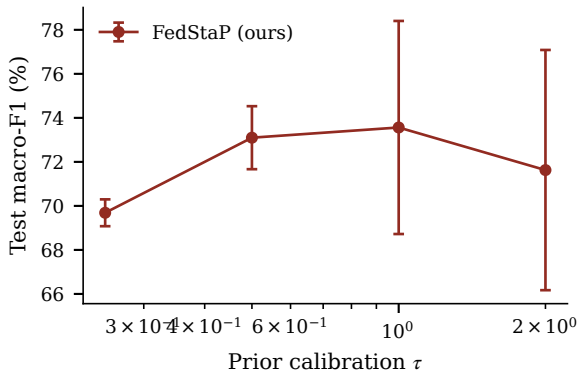
Edge-IIoTset
