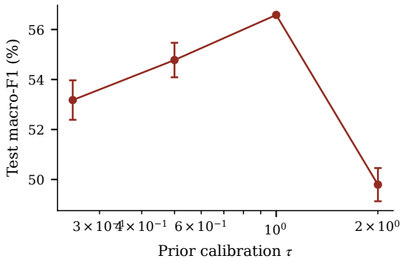
CICIoT2023
