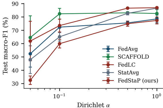
Edge-IIoTset
